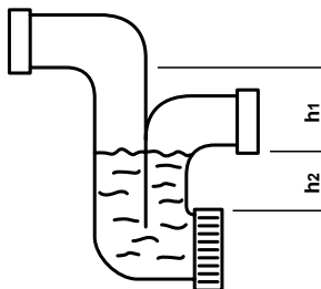
Обычный сифон
