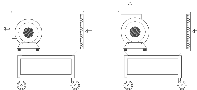
ВАРИАНТ МОБИЛЬНОЙ УСТАНОВКИ
